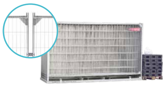
Mobile Secure Reinforced Artnr. KIT 105M 02 1st Transportpall 30st Mobile Secure 3,5m förstärkta 30st Demex 20kg fundament 30st kopplingsklammer 0,5kg
