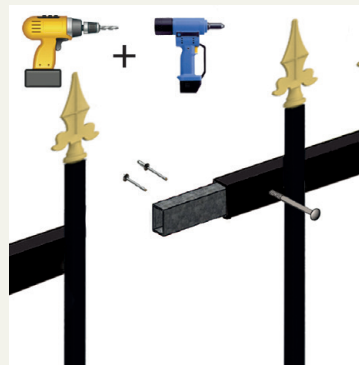
2 trous de Ø4,2mm 2 rivets
