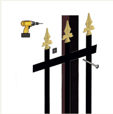
2 trous de Ø8,5mm 2 vis à tête plate m8 x 110
