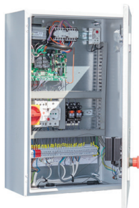
Styrskåp
