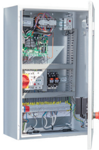
Styrskåp
